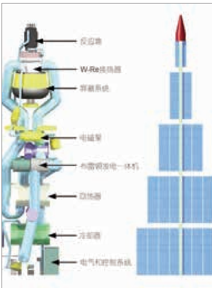
Esquema del prototipo de reactor nuclear refrigerado por litio.
