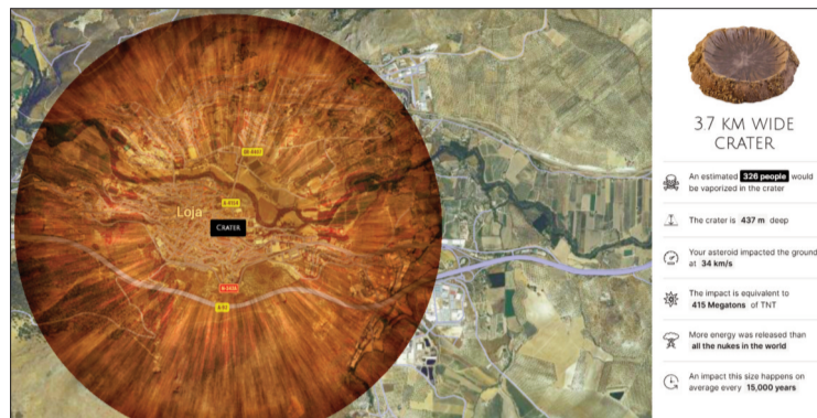
Simulación del impacto de un asteroide en Loja
